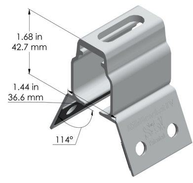
RibBracket™ IV
