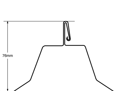
76mm Trap Snap Seam S-5-V, S-5-V Mini S-5-U, S-5-U Mini
