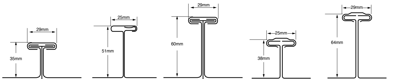
35mm T Seam S-5-T, S-5-T Mini
