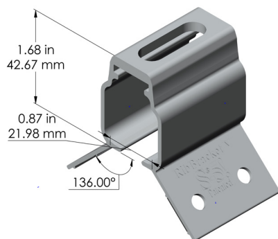
RibBracket™ II
