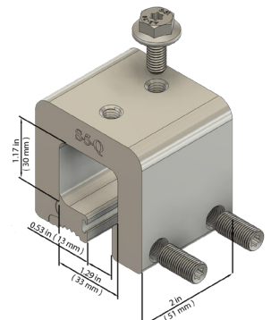
S-5-Q™
