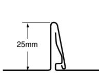
25mm Snap Seam S-5-S, S-5-S Mini
