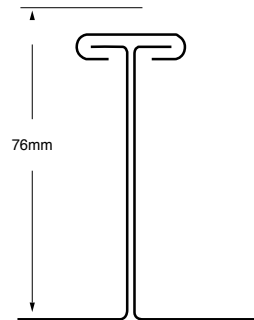
76mm Batten Cap T Seam S-5-T, S-5-T Mini
