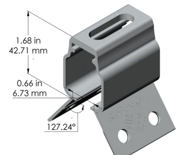
RibBracket™ I
