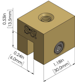
S-5-B™ Mini
