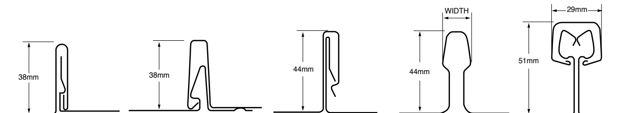
38mm Snap Seam S-5-S, S-5-S Mini
