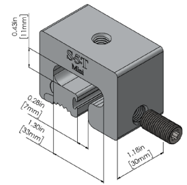
S-5-T™ Mini
