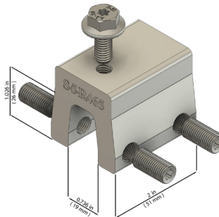
S-5-R465™
