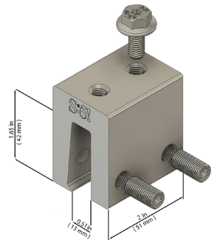
S-5-N 1.5™
