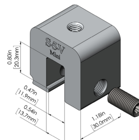
S-5-V™ Mini
