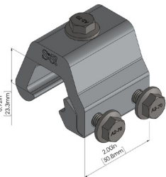
S-5-K Grip™ Mini
