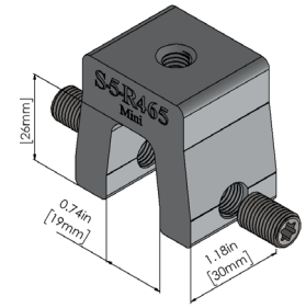
S-5-R465™ Mini
