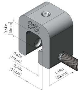
S-5-MX™ Mini
