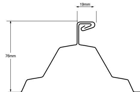
76mm Trap Single Fold S-5-H90, S-5-H90 Mini S-5-U, S-5-U Mini S-5-H, S-5-H Mini
