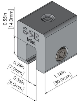
S-5-E™ Mini
