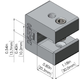
S-5-H90™ Mini
