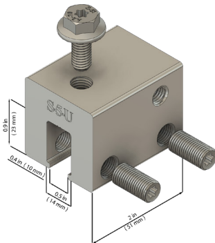
S-5-U™
