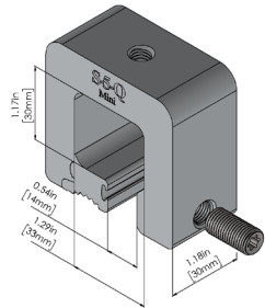
S-5-Q™ Mini
